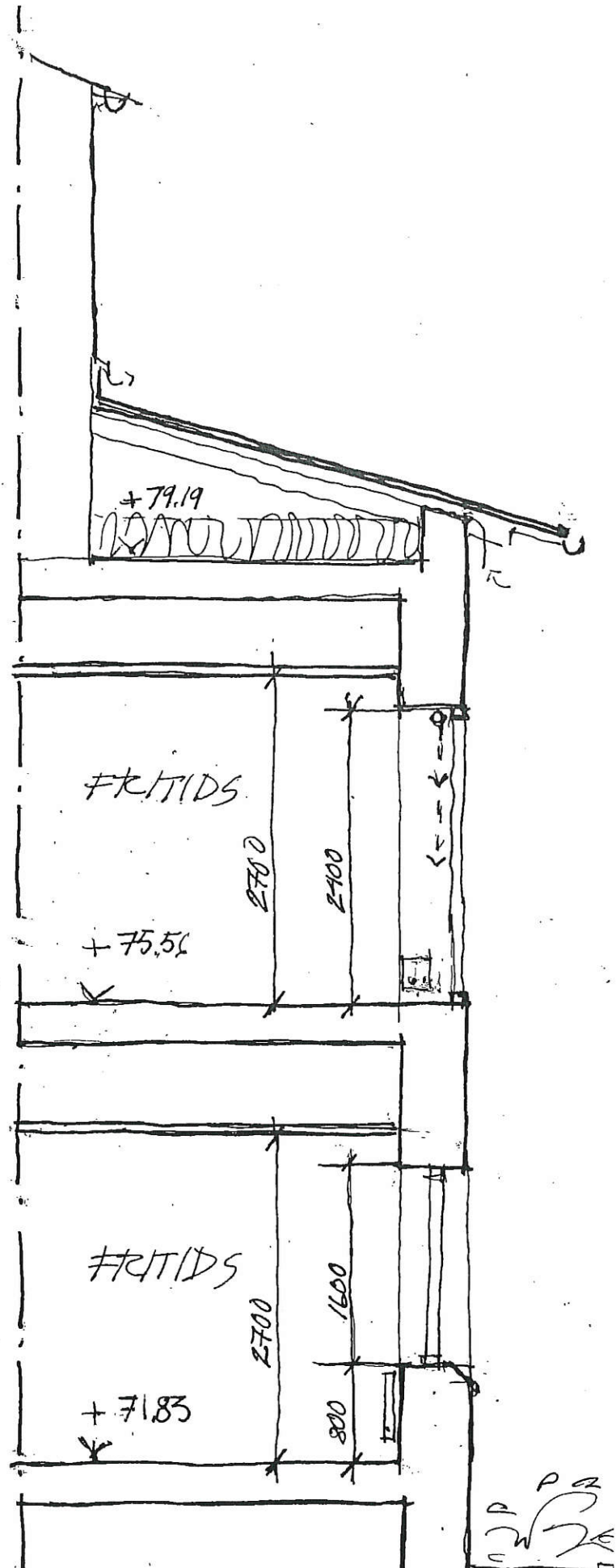
SEKTION A-A
